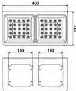
LED- 三菱 / 日野货车尾灯 ( 不锈钢两格 ) LED TAIL LAMP
