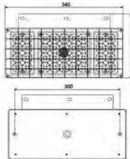
LED- 铁制 - 五十铃后尾灯 - 黑 LED TAIL LAMP
