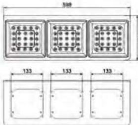
LED- 三菱 / 日野货车尾灯 ( 不锈钢三格 ) LED TAIL LAMP
