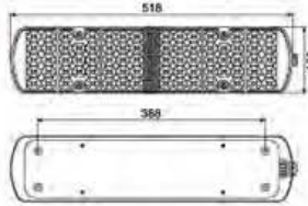
LED- 奥威后尾灯 ( 塑制 ) 适用于二三吨后尾灯 LED TAIL LAMP
