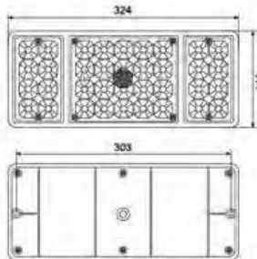
LED- 东风 140-2 后尾灯 II 型 LED TAIL LAMP
