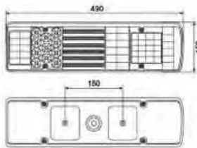
LED- 德龙 / 奥龙后尾灯 LED TAIL LAMP
