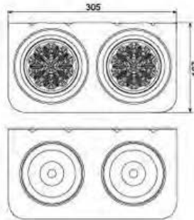
LED- 中集挂车橡皮后尾灯 - 双体 LED TAIL LAMP
