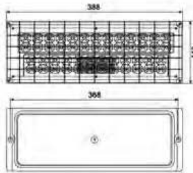
LED- 新江淮 153 后尾灯 - 黑 LED TAIL LAMP
