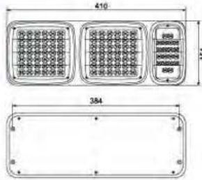
LED- 巨能王水晶后尾灯 I 型 LED TAIL LAMP
