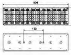
LED- 高亮斯太尔王铁制后尾灯 (封闭式防水型, 带网罩) LED TAIL LAMP
